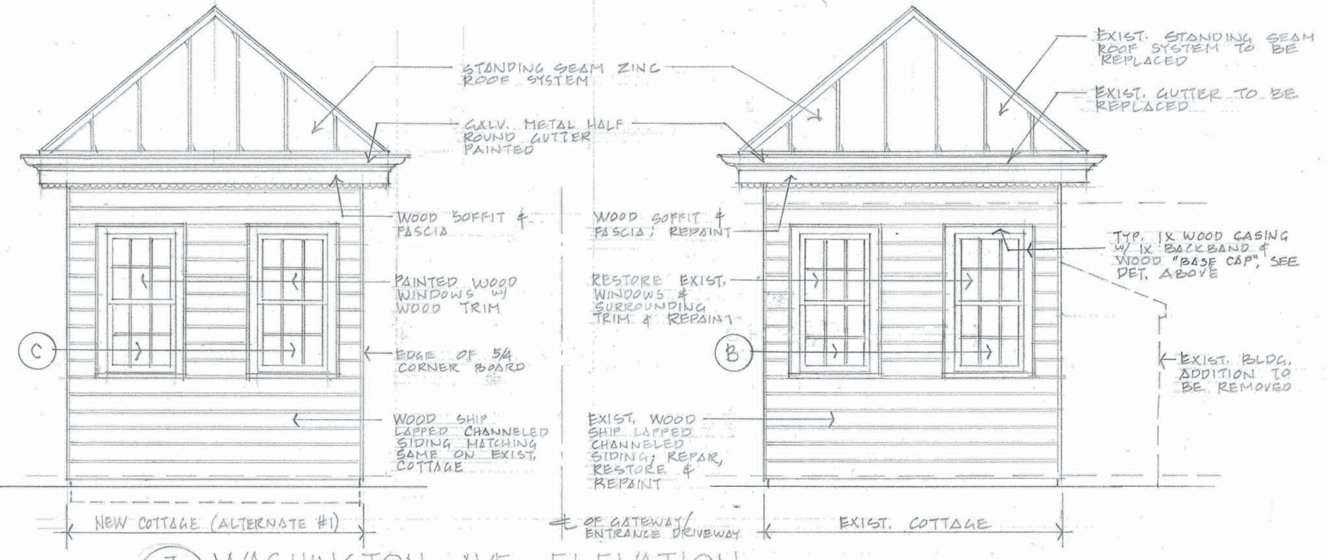
7 WASHINGTON AVE. ELEVATION SCALE: 1/4" = 1'-0"
