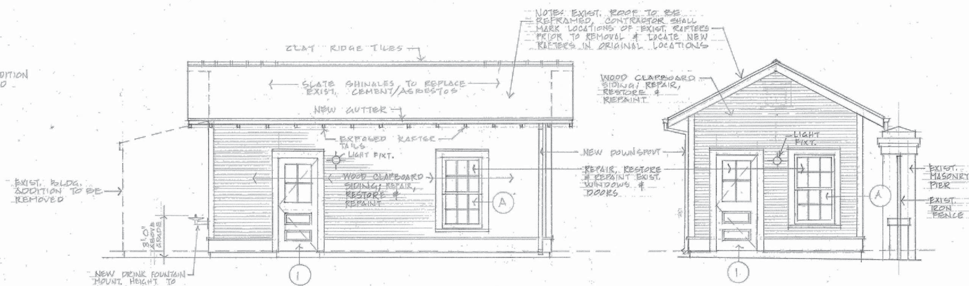
6 WASHINGTON AVE. (SIDE) ELEVATION A1 SCALE: 1/4" = 1'-0"
