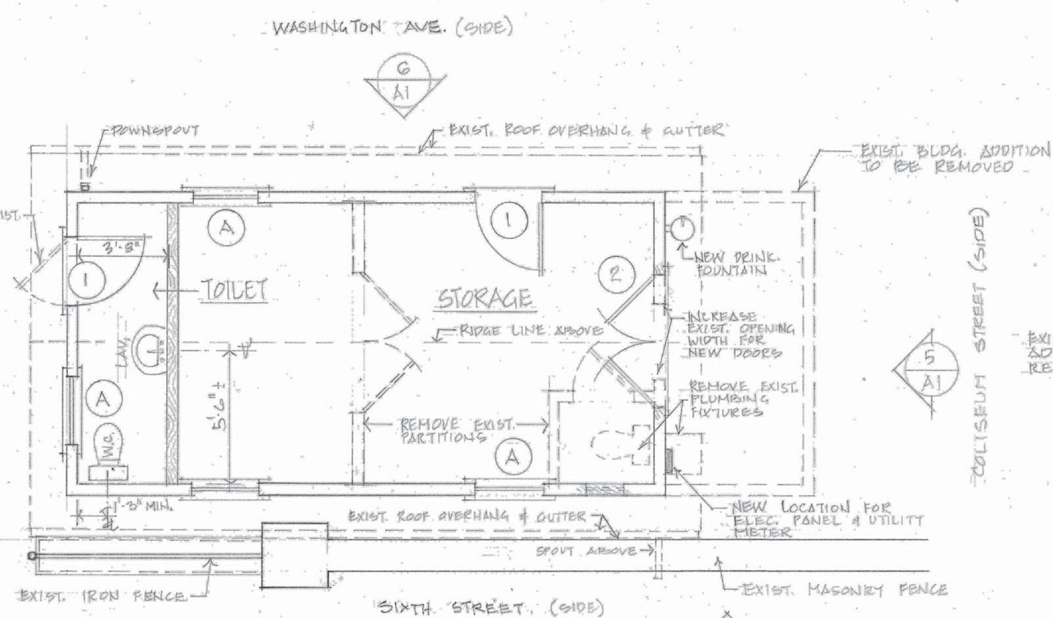
2 FLOOR PLAN A1 SCALE: 1/4" = 1'-0"
