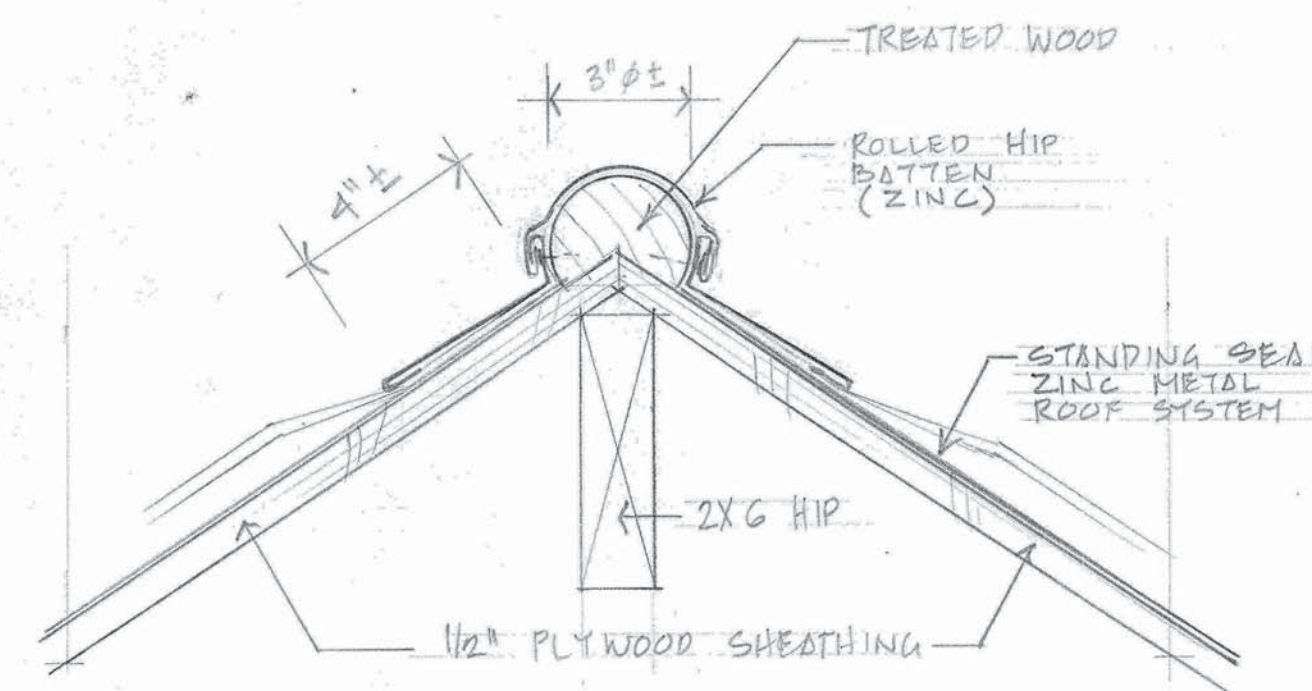
1 HIP DETAIL SCALE: 3"=1'-0"
