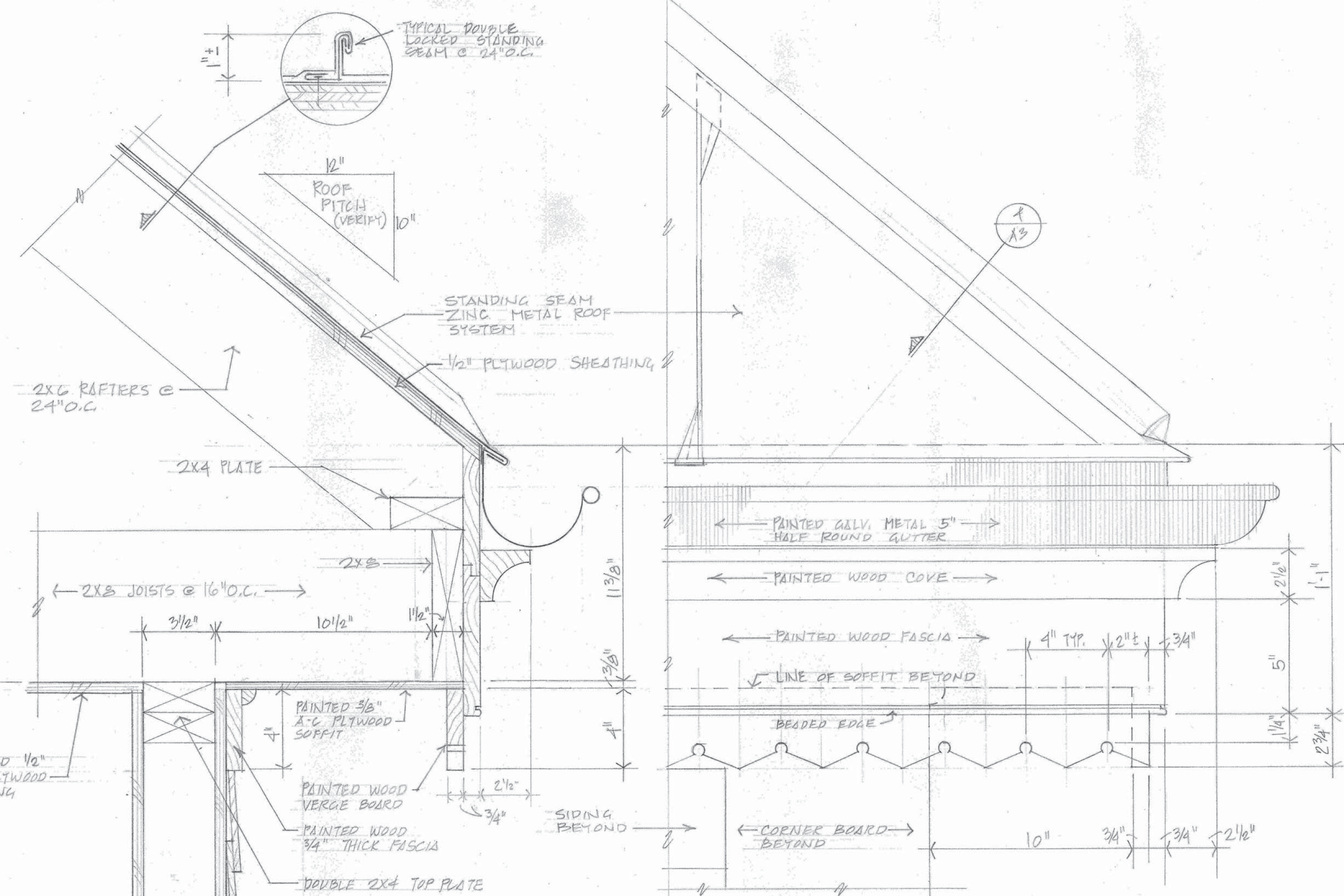
2 CORNICE ELEVATION DETAIL SCALE: 3"=1'-0"
